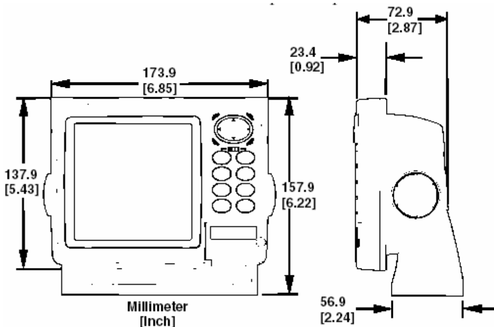
Монтаж X47EX на держателе. Вид спереди (слева) и сбоку (справа)
